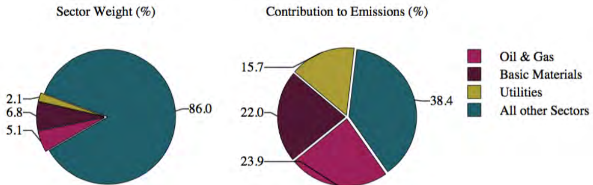
Abbildung 5: Sektoren-Betrachtung (Fondsmarkt)
